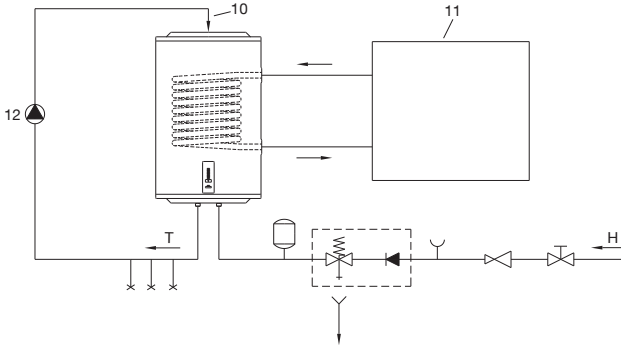
4 Сурет: Балама жылыту көздеріне жалғау
