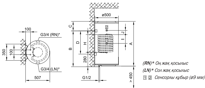
1 Сурет: Қабырғаға сатылас түрде жинақтау
