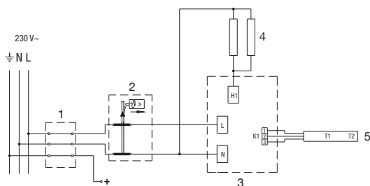
Рисунок 6: Электросхема
