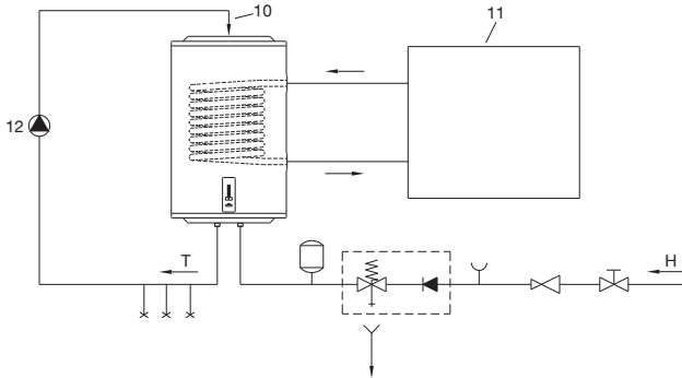
SI. 4: Priklučivanje na druge izvore grejanja
