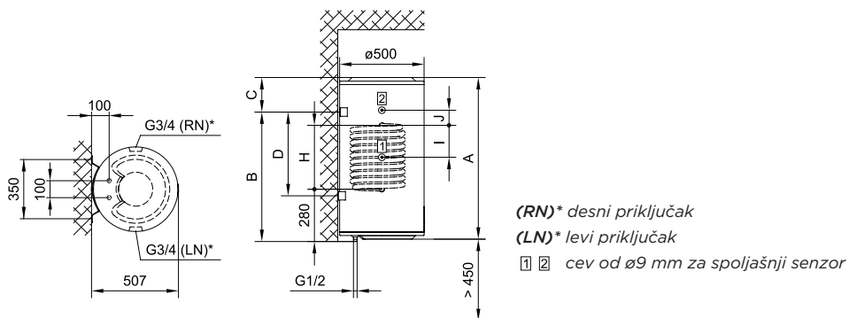
Sl. 1: Vertikalno montiranje na zid
