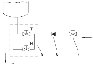
Fig. 3: Sistemul deschis (nepresurizat)
