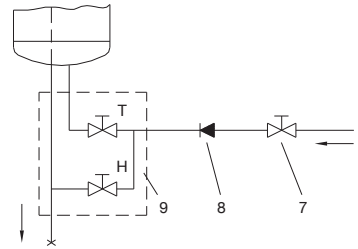
3 Сурет: Қысымсыз (ашық) жүйе
