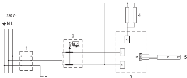
6 Сурет: Электрсхемасы
