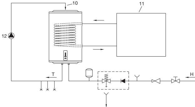
Fig. 4: Conectarea încălzitorului la sursa de energie suplimentară.
