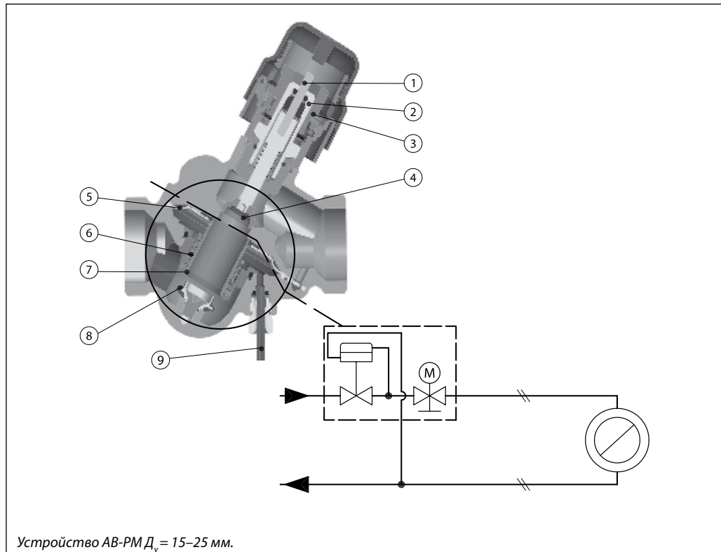
Устройство АВ-РМ Д у = 15–25 мм.
