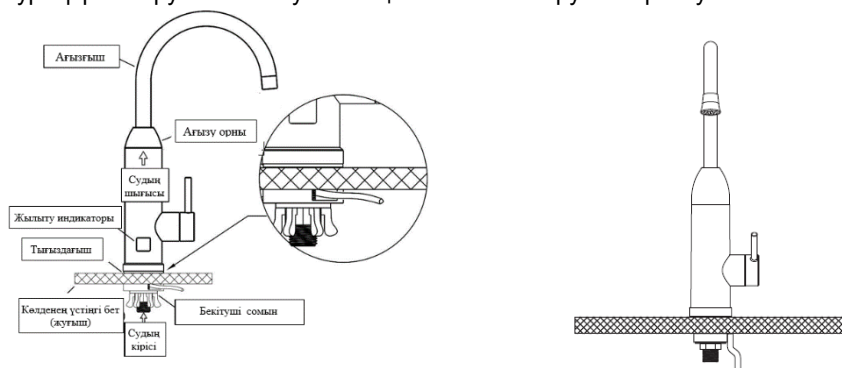
2-сур. Қорек беру кабелін жуғыштың астынан шығарумен орнату
